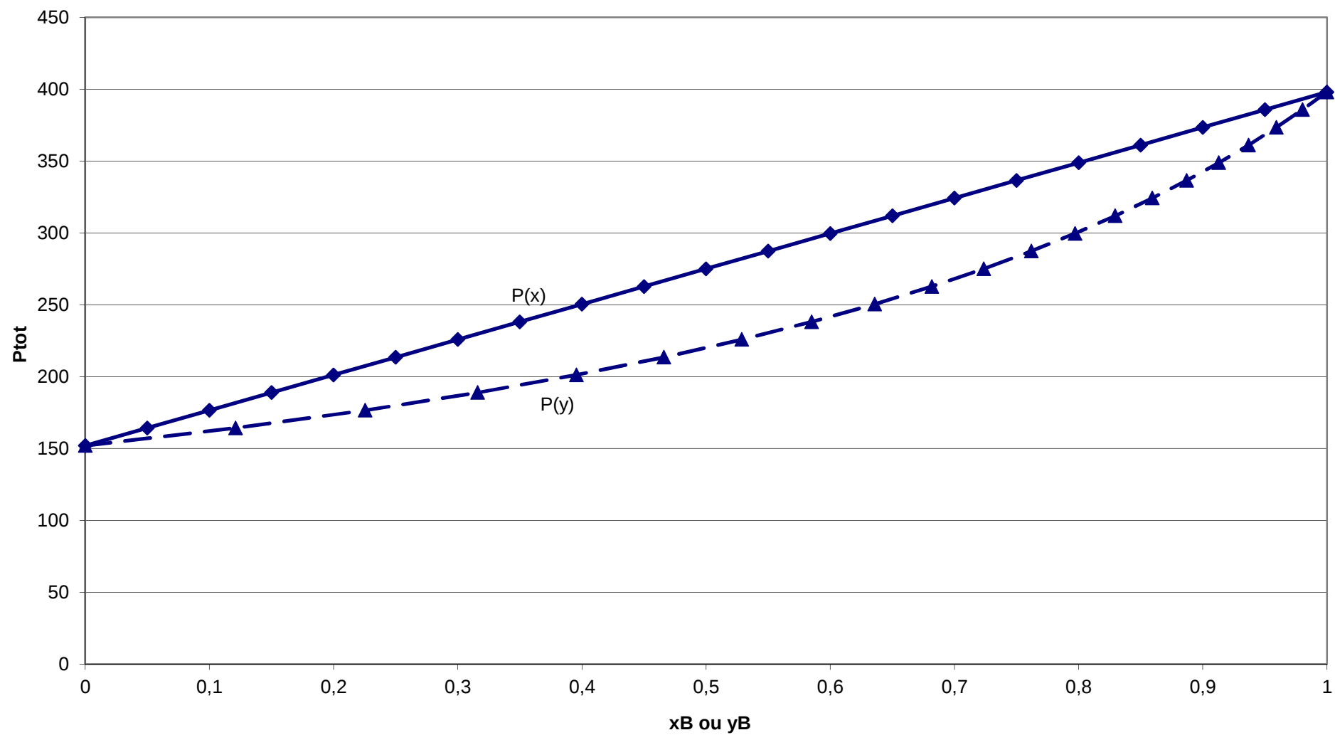
isotherme benzène-toluène à 60°C (ex n°4 du doc potentiel chimique)
